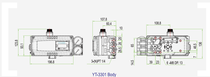
YT-3301 Body
